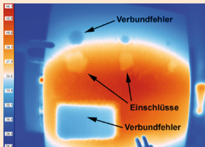
Wärmefluss-Thermographie einer Sandwichplatte mit Aluminium-Wabenkern
