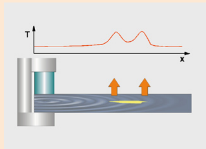
Prinzip der Dunkelfeldthermographie
