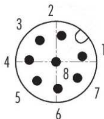
M12A
